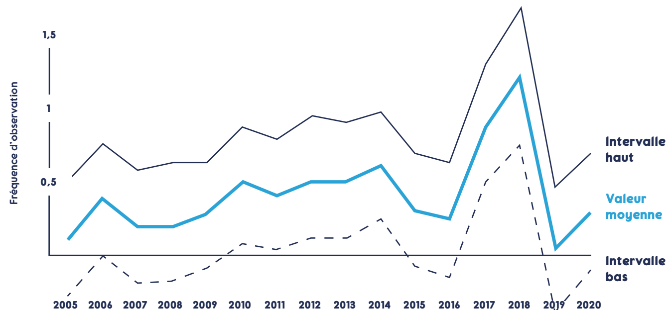
Fréquence d'observation modélisée sur la base des données 2005-2018 et prédictions pour les années 2019 et 2020
